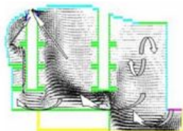
FLUJO DE VENTILACIÓN UPC
